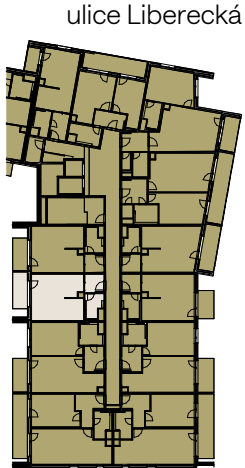
Přehled ploch
